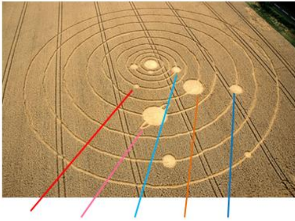
Mars Saturn Earth Jupiter Uranus
